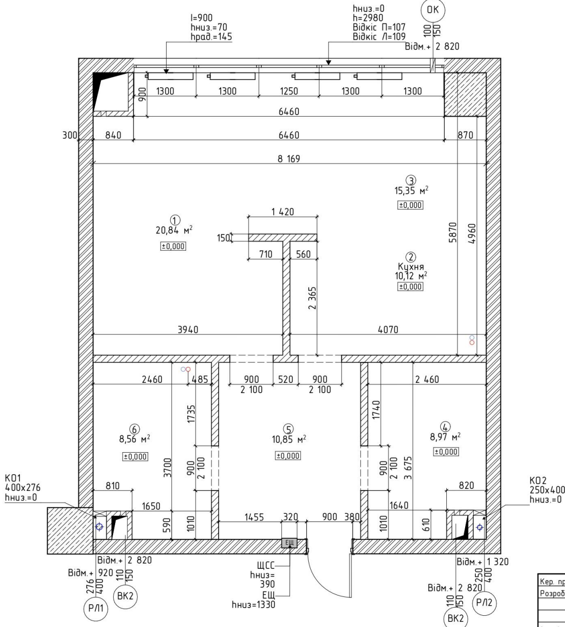
Обмірний план М 1:50
