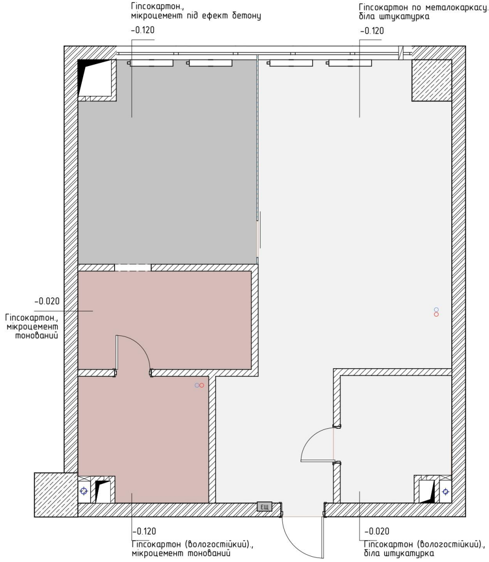
План стелі М 1:50
